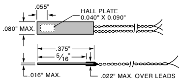
Model BH-205 Mini Transverse
