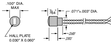
Model BH-204 Mini Axial
